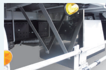
●独立保護板 ステンレス製
