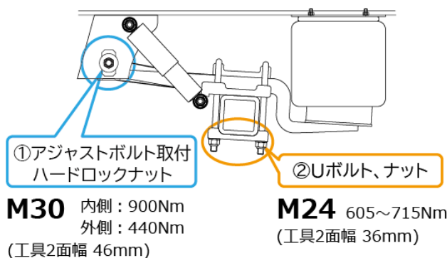
M30アジャストボルトの例
