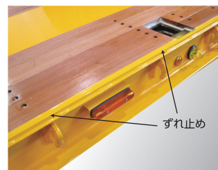
●床板二重張り ずれ止め有
