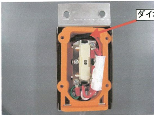
(羽根開閉スイッチ内部)
