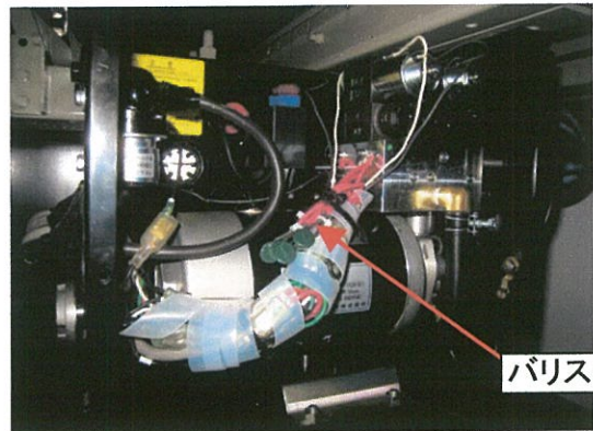
(パワーユニット内部)
